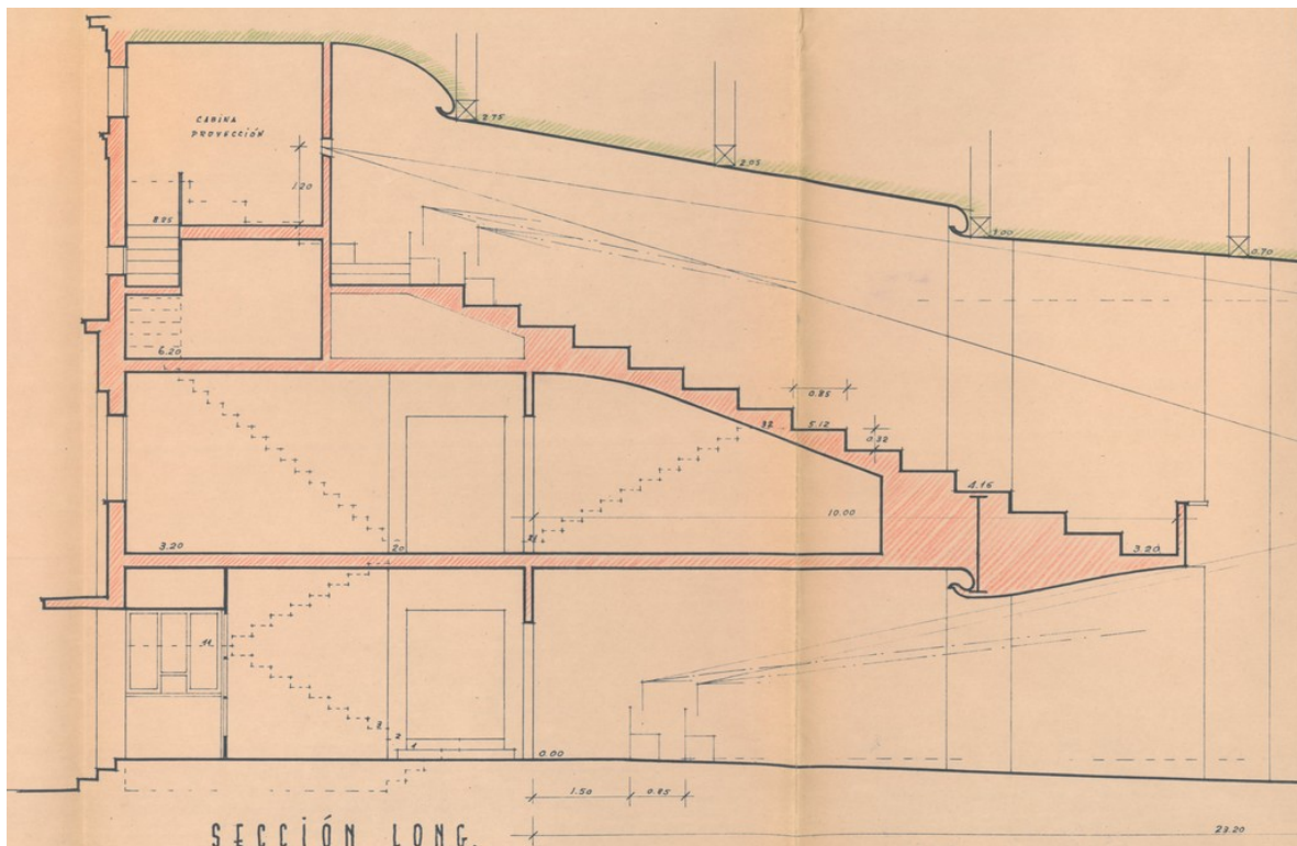
Fragment del plànol de secció longitudinal
