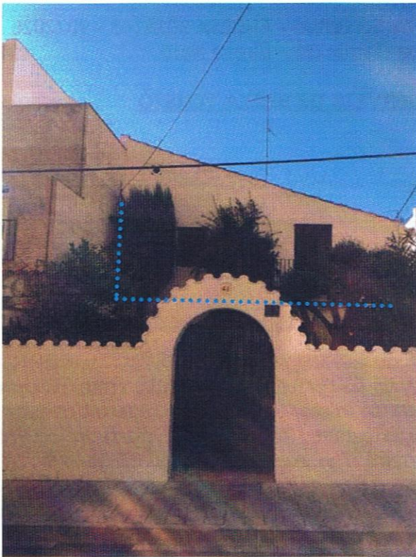
Foto 1: Detall traçat escomesa B.T. aèria . (Escomesa grapada a façana sota tub des de punt de connexió actual fins a CDU en vorera, en el límit en façana )
