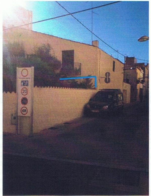
Foto 1: Detall traçat escomesa B.T. aèria . (Escomesa grapada a façana sota tub des de punt de connexió actual fins a CDU en vorera, en el límit en façana )
