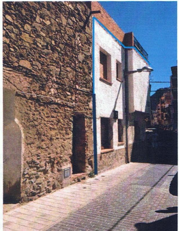
Foto 2: Detall traçat línia B.T. trenada i conversió A/S.
