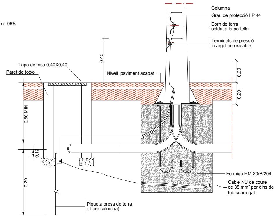
FONAMENT COLUMNA TIPUS I PICA
