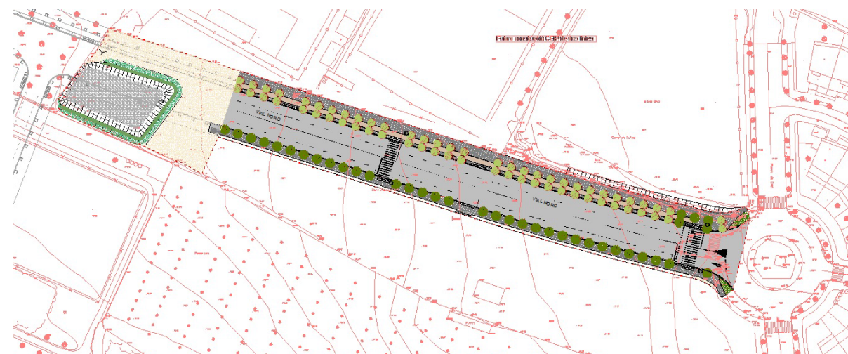
Figura.- Planta general de les obres d'urbanització
