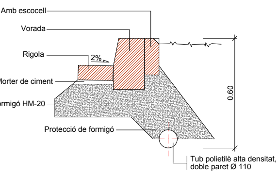
PROTECCIÓ CONDUCCIÓ ENLLUMENAT AMB FORMIGÓ
