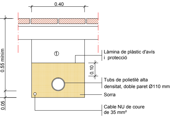
RASA TIPUS PER A ENTUBAR CABLES A ZONA DE VORERES
