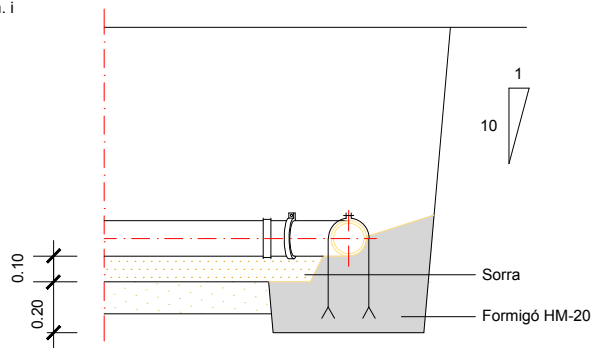
ANCORATGE
