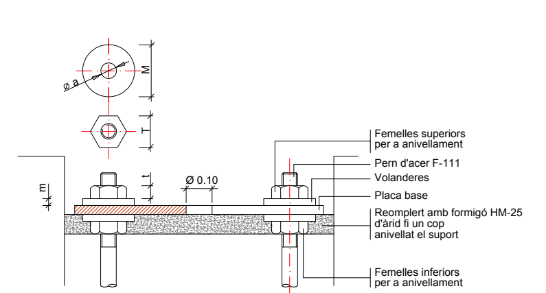
Detall ancoratges de les columnes i bàculs
