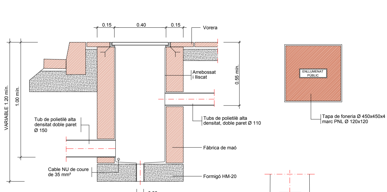
ARQUETA TIPUS I TAPA
