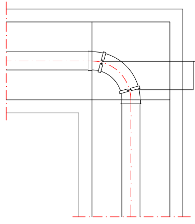
PLANTA DERIVACIÓ A 90° (COLZE)
