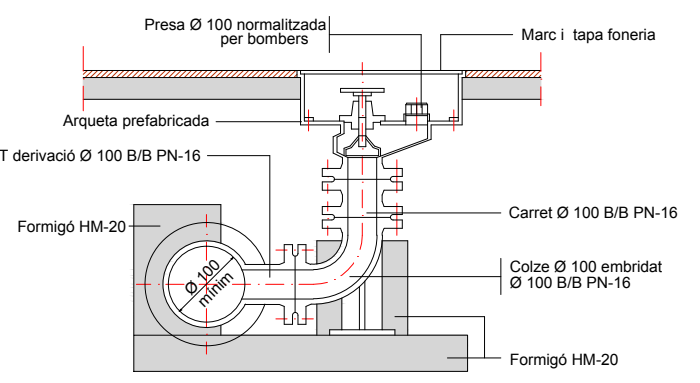
HIDRANT SOTERRAT
