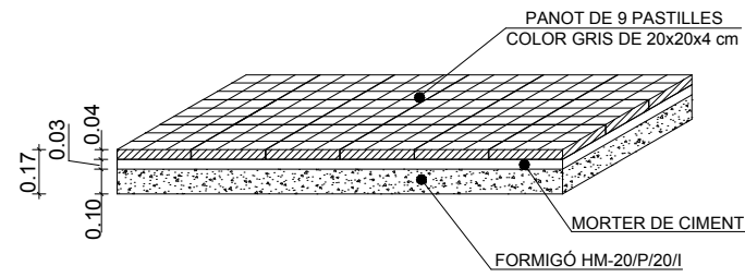
PAVIMENT DE PANOT S/E
