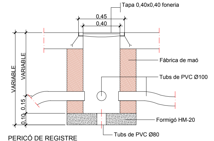
PERICÓ DE REGISTRE
