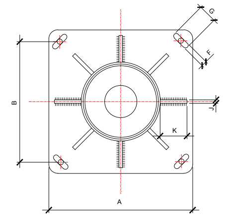
SECCIÓ A-A'
