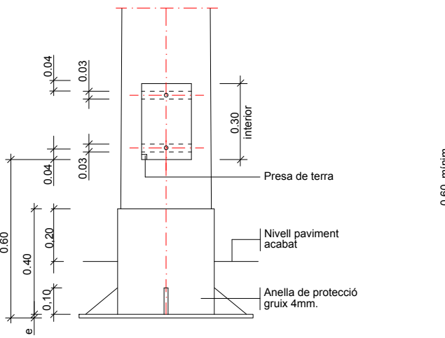
Columna i plaques base DETALL COLUMNA I EMPOTRAMENT EN PAVIMENT
