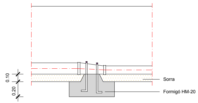
ANCORATGE
