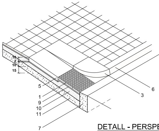
DETALL - PERSPECTIVA
