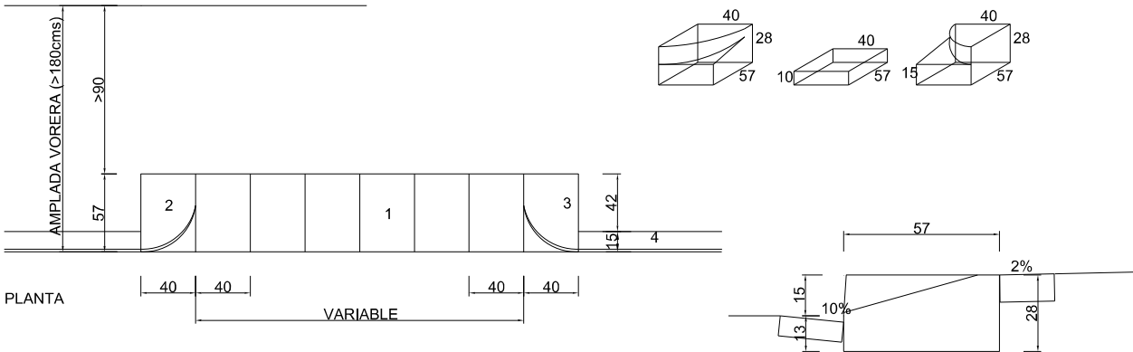
GUAL VEHICLES TIPUS 1
