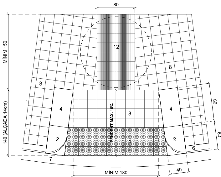
GUAL ACCESSIBLE VIANANTS TIPUS 2
