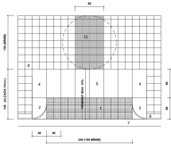
GUAL ACCESSIBLE VIANANTS TIPUS 1
