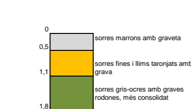
Nº PENETROMETRE: P-10 (9,5m) Nº TALL SOBRE P-10 cota 11,3m
