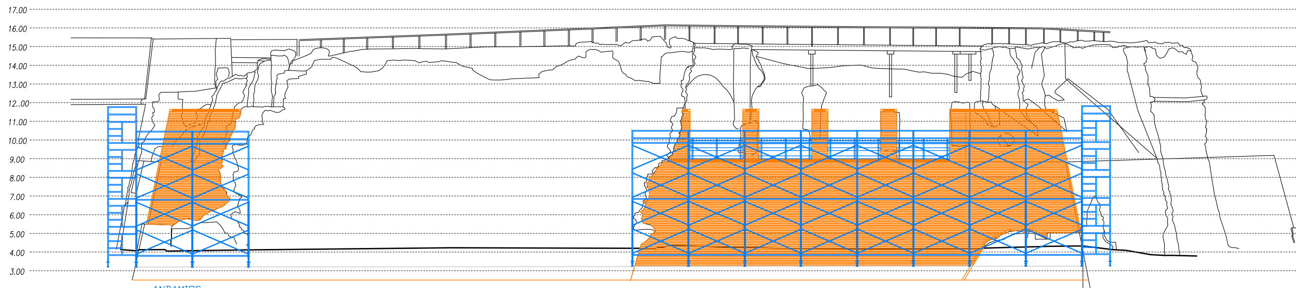
BARANDILLAS EN PROTECCIÓ DE CAIDAS VERTICALES, Se colocaran durante la ejecuci3n del pavimento y coronaci3n entre los contrafuertes
