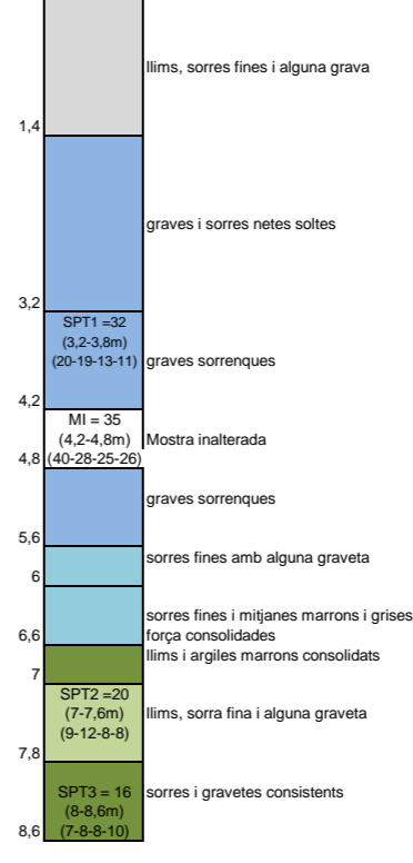
SONDEIG S-1 (P4)
