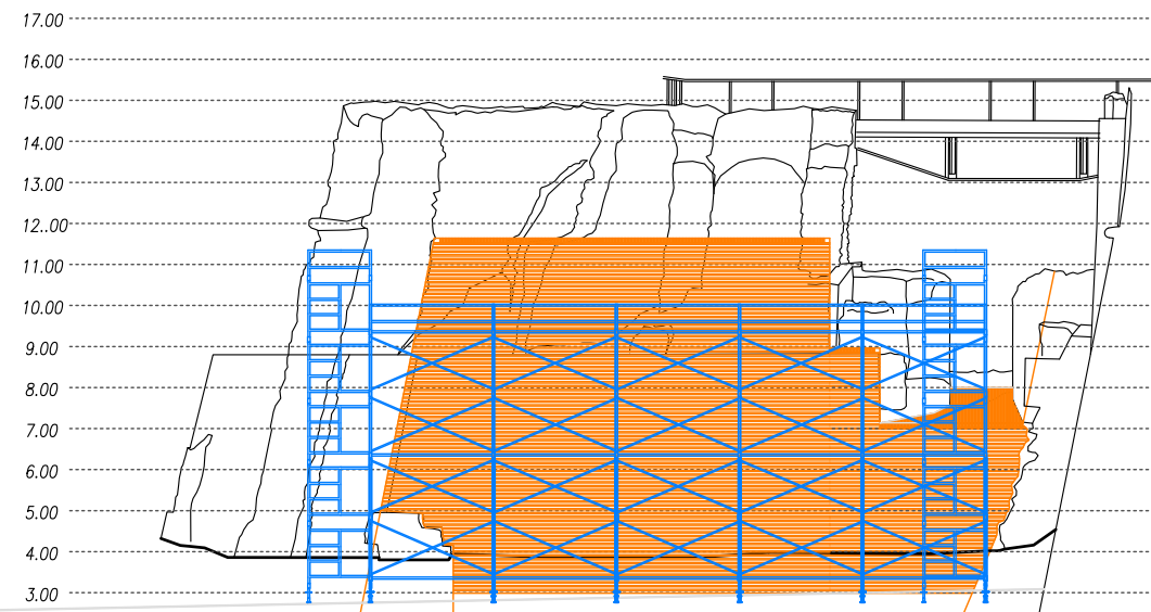
ALZADO OESTE ANDAMIOS Se utilizaran durante los trabajos de paletteria y revestimientos de fachada y pavimentos, entre los lienzos. Los andamios tendran que llevar barandillas y escaleras con trampillas, y se colocaran sobre una base estable y tolerable.
