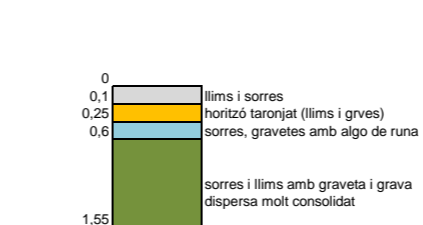
Nº PENETROMETRE: P-12 (8m) Nº TALL SOBRE P-12 cota 9,5m
