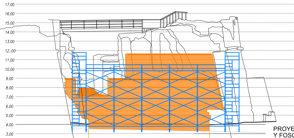
ALZADO SUR BARANDILLAS EN PROTECCIÓ DE CAIDAS VERTICALES, Se colocaran durante la ejecuci3n del pavimento y coronaci3n entre los contrafuertes
