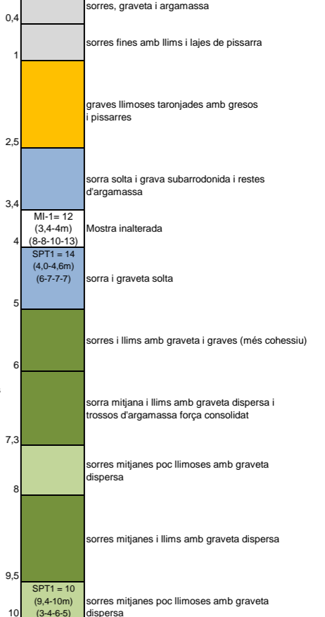
SONDEIG S-2 (P7)
