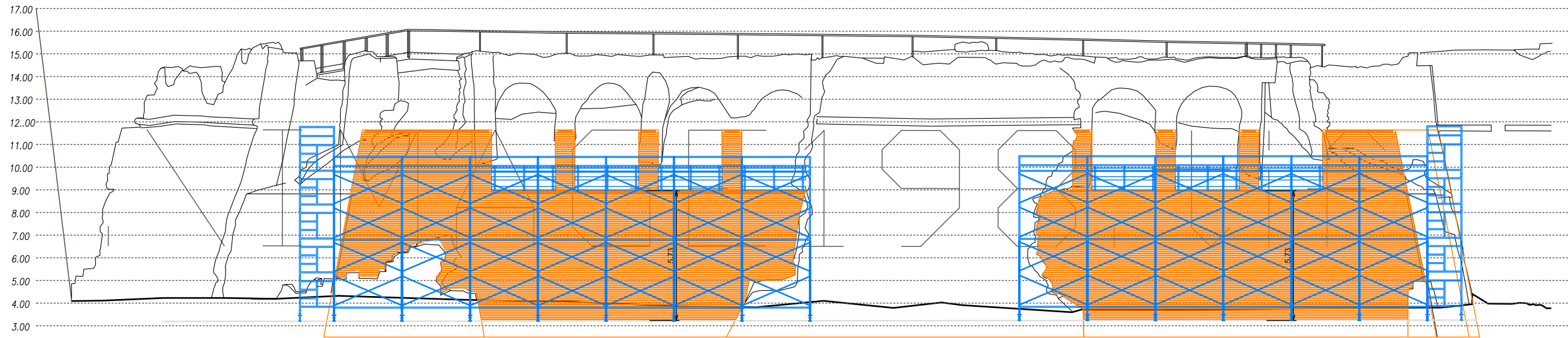
ALZADO NORTE ANDAMIOS Se utilizaran durante los trabajos de paletteria y revestimientos de fachada y pavimentos, entre los lienzos. Los andamios tendran que llevar barandillas y escaleras con trampillas, y se colocaran sobre una base estable y tolerable.
