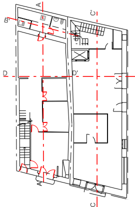
PLANTA BAIXA
