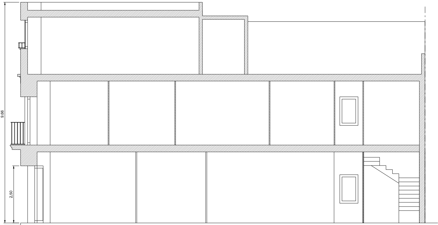
ALÇAT-SECCIÓ C-C'
