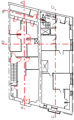
PLANTA PRIMERA
