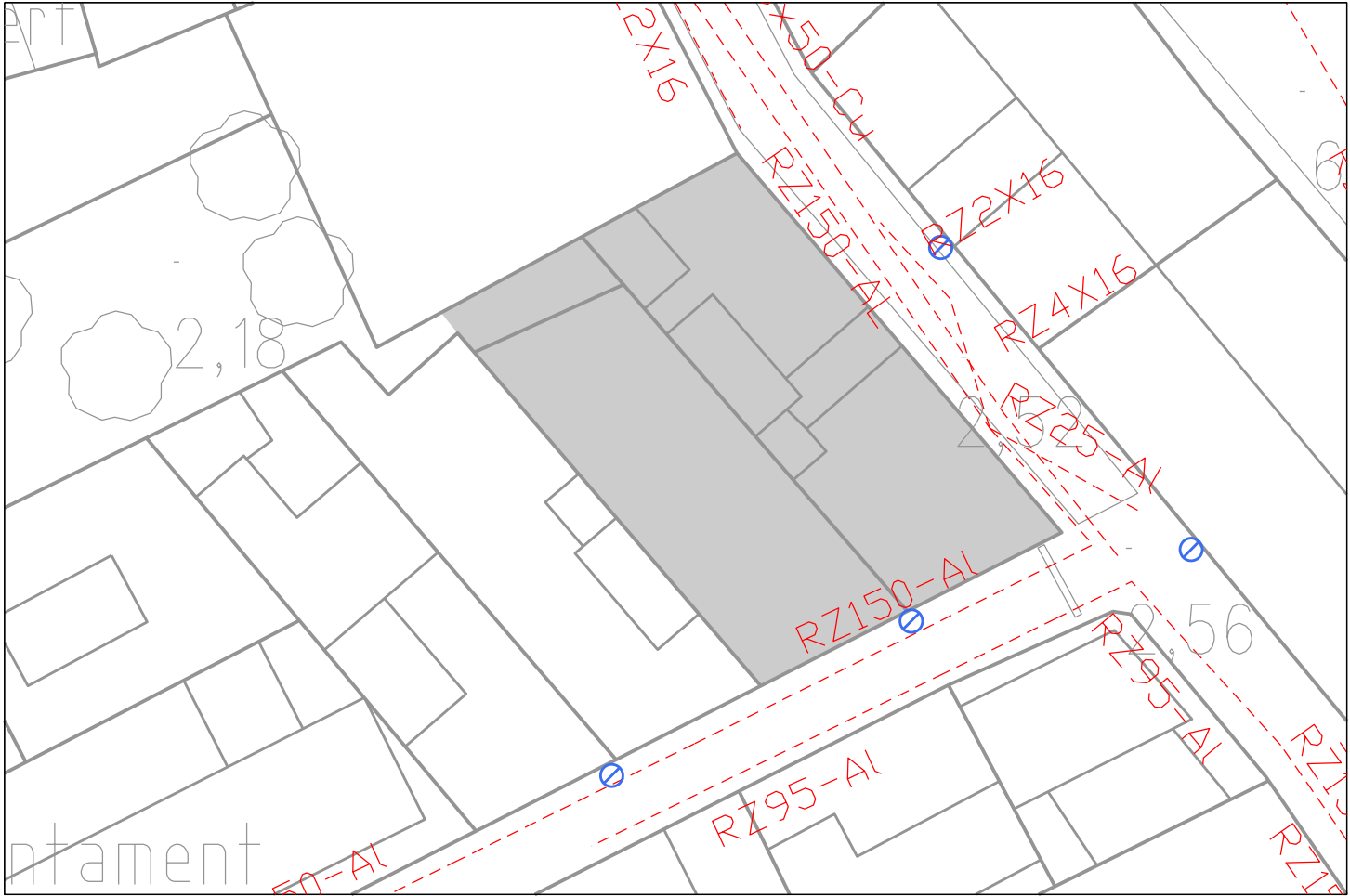
XARXA ELECTRICITAT I ENLLUMENAT PÚBLIC
