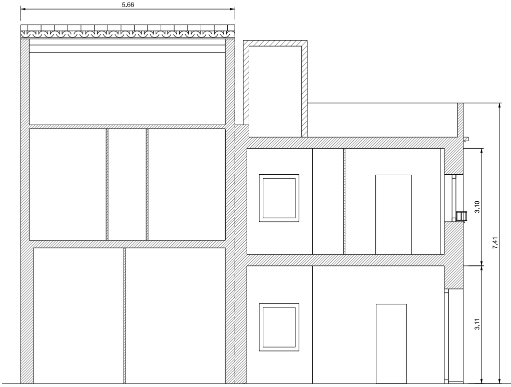
ALÇAT-SECCIÓ D-D'
