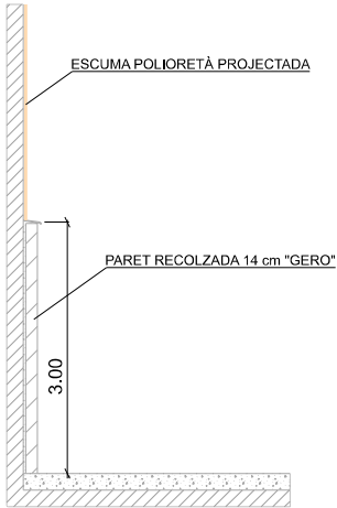
DETALL PARET RECOLZADA A MITGERA
