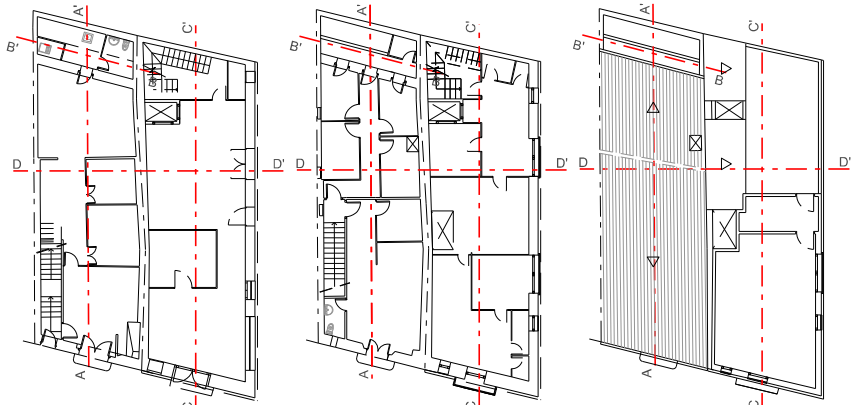
PLANTA BAIXA
