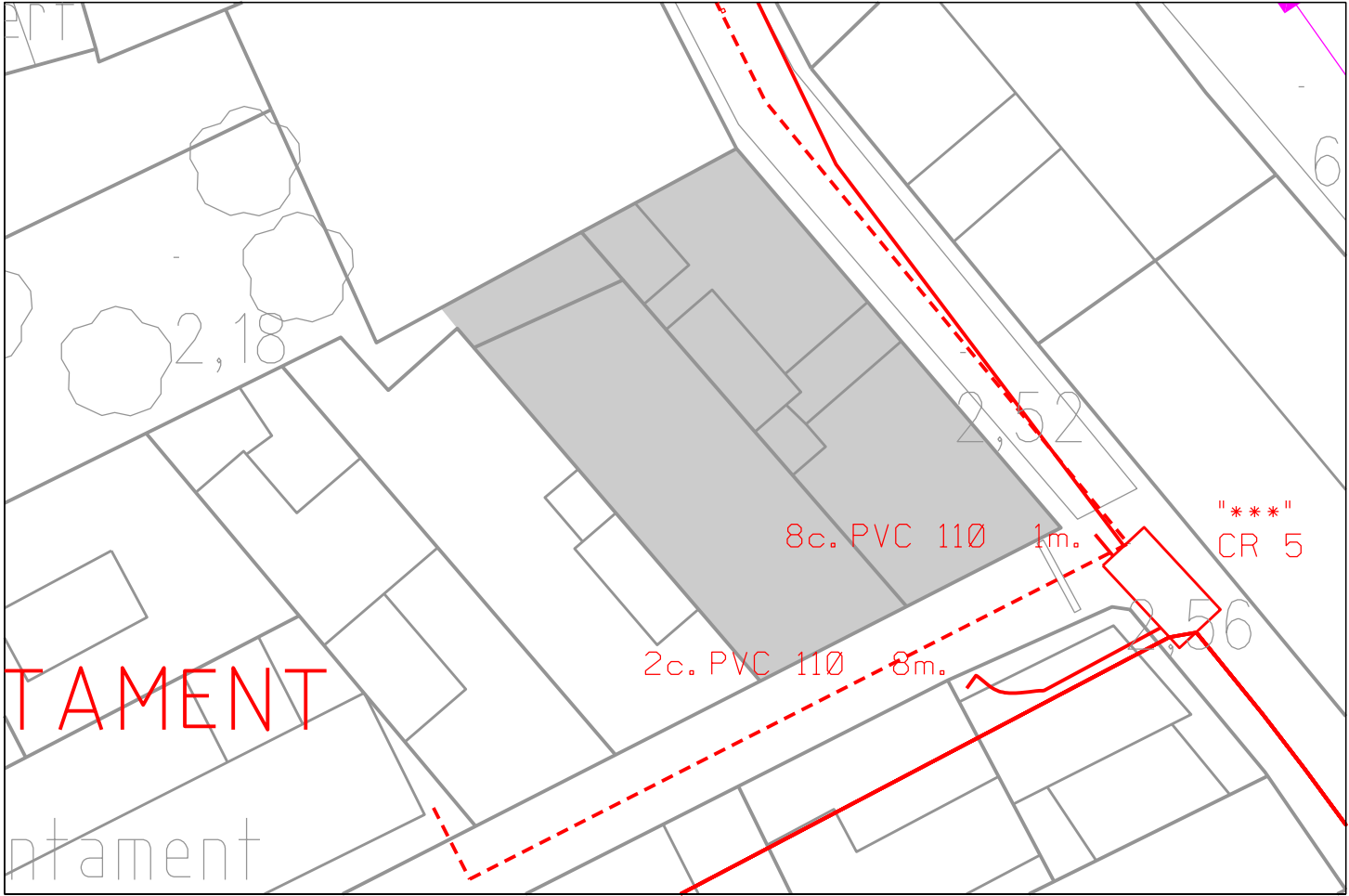
XARXA TELÈFON I TELECOMUNICACIONS
