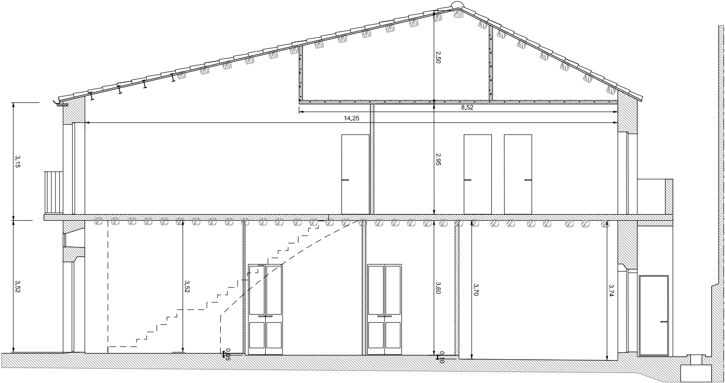
ALÇAT-SECCIÓ A-A'
