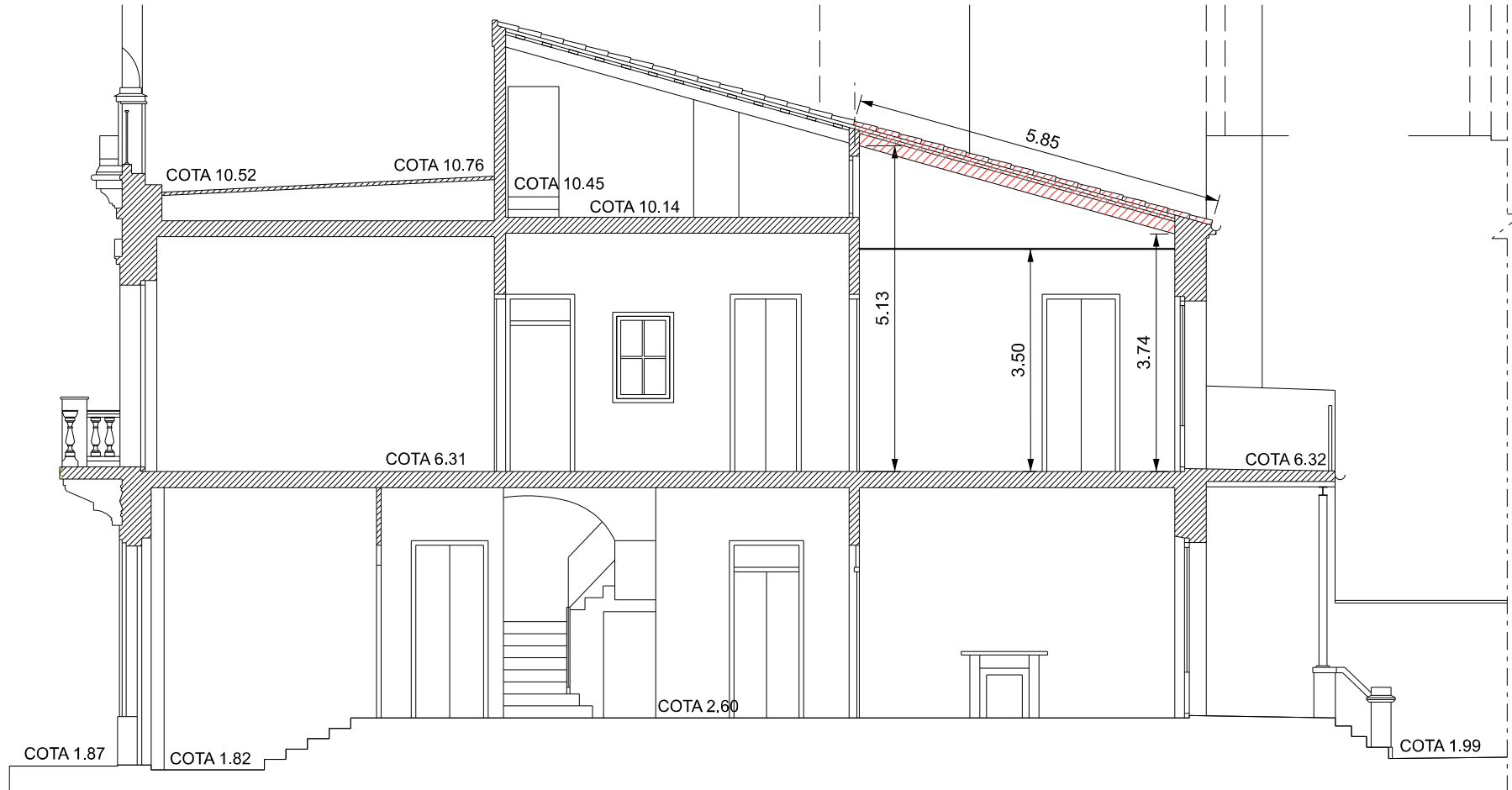
SECCIÓ A-A'
