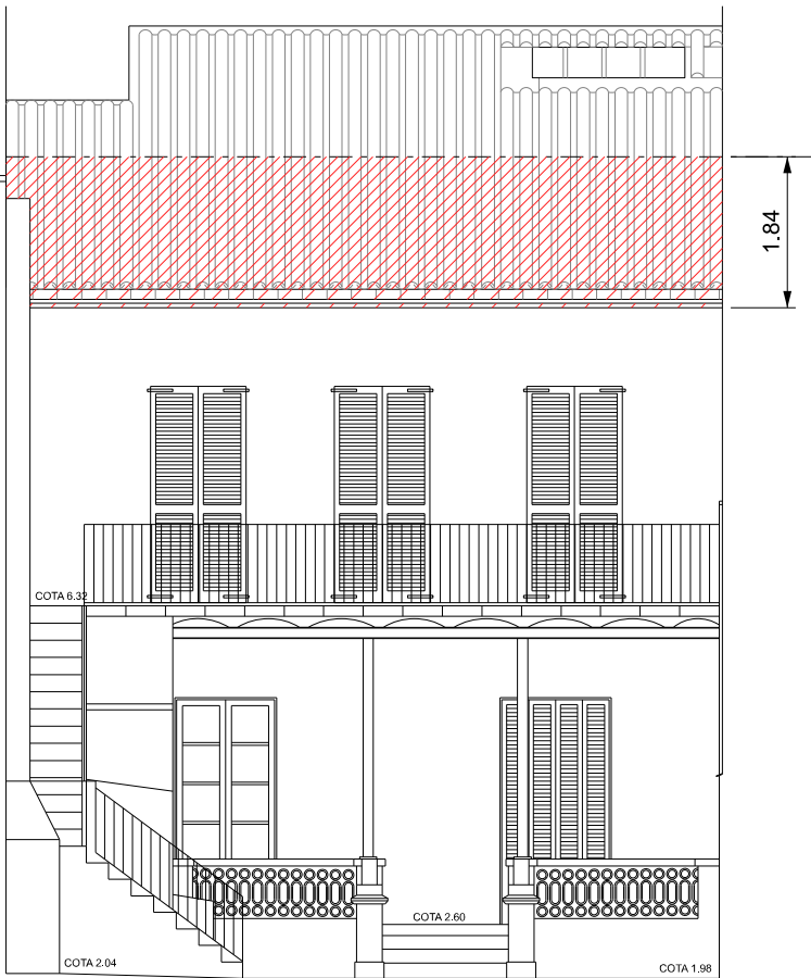
FAÇANA INTERIOR
