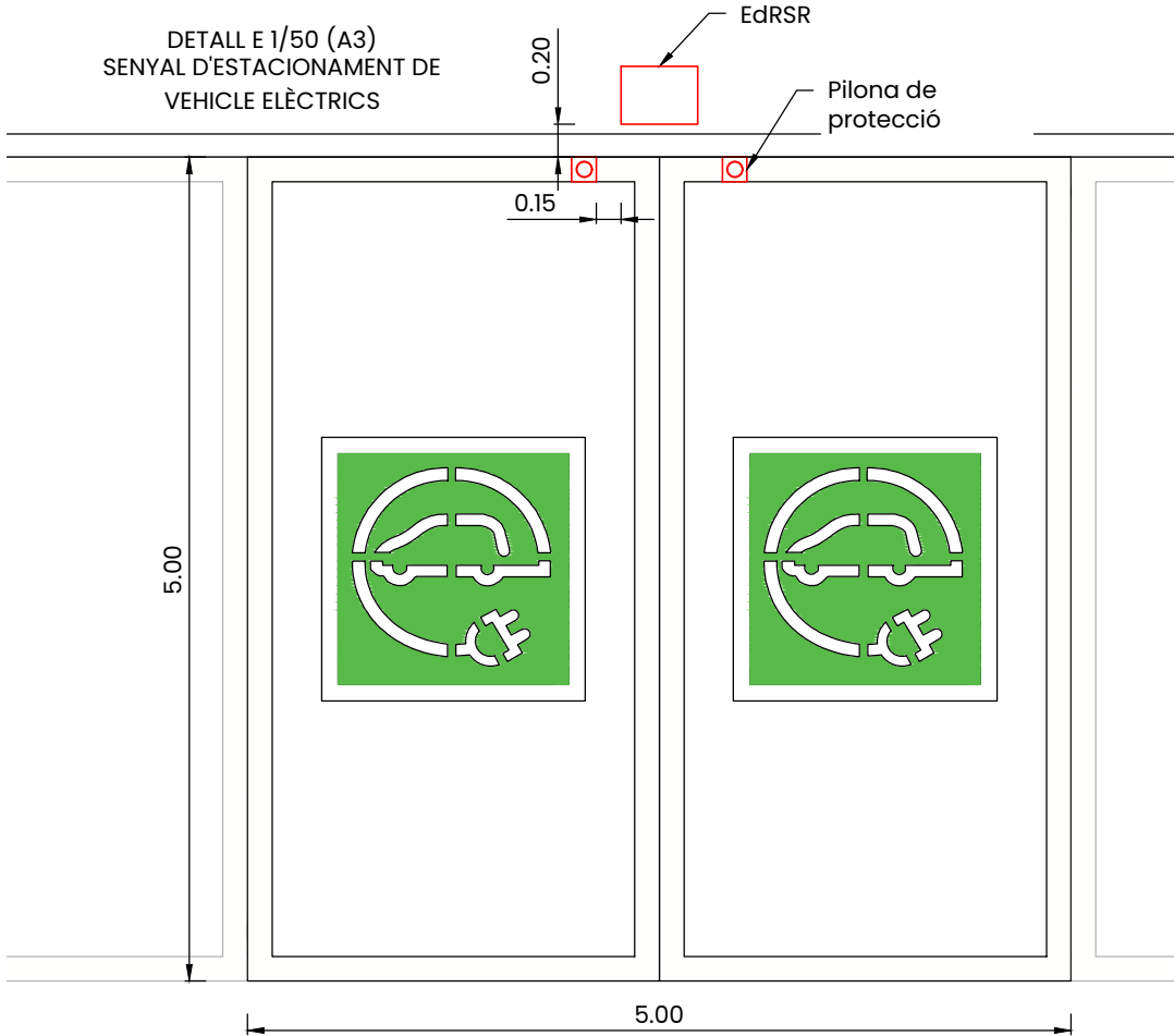
DETALL E 1/50 (A3) PINTURA DE PLAÇA DE VE SEGONS INSTRUCCIÓ MOV 2022/12
