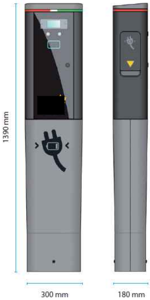
DETALL E 1/20 (A3) DE L'EdRSR 20+20 kW
