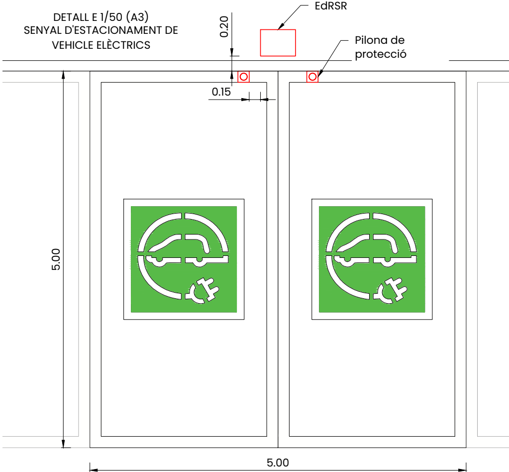
DETALL E 1/50 (A3) PINTURA DE PLAÇA DE VE SEGONS INSTRUCCIÓ MOV 2022/12
