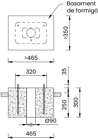
DETALL E 1/20 (A3) BASAMENT DE L'EdRSR
