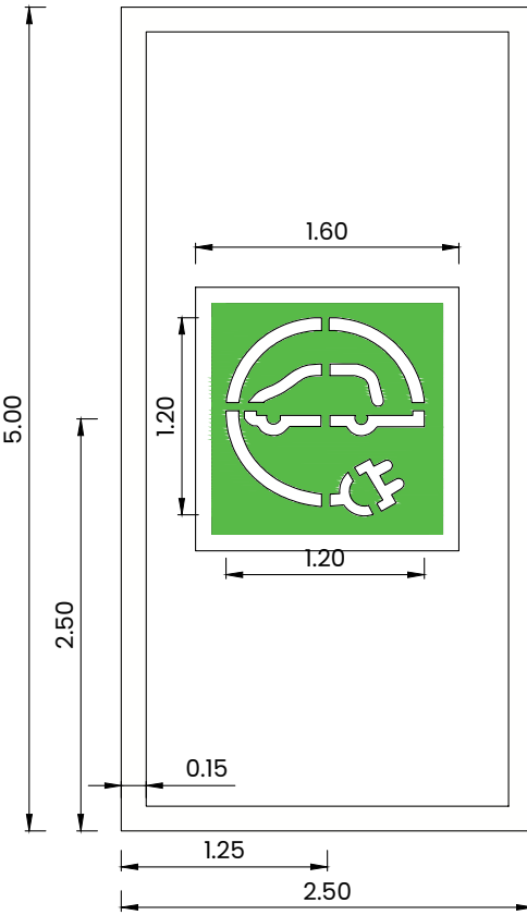
DETALL E 1/50 (A3) PINTURA DE PLAÇA DE VE SEGONS INSTRUCCIÓ MOV 2022/12
