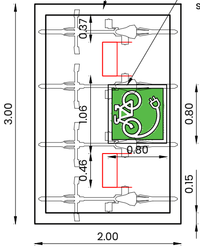
Aparcament per a dues bicicletes elèctriques Orientació del símbol segons plànols 2 i 3
