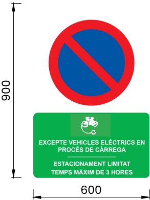
DETALL E 1/20 (A3) SENYAL D'ESTACIONAMENT DE VEHICLE ELÈCTRICS
