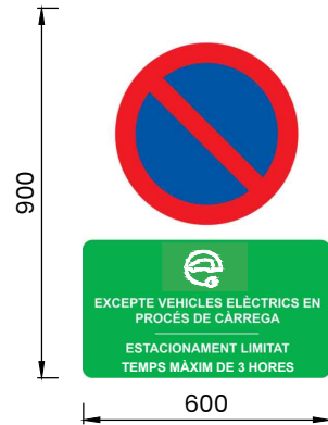
DETALL E 1/20 (A3) BASSAMENT SENYAL
