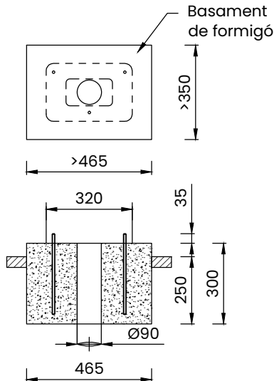
DETALL E 1/20 (A3) BASAMENT DE L'EdRSR
