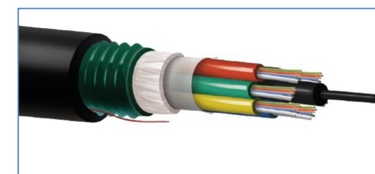
Estructura de la mànega multitub
