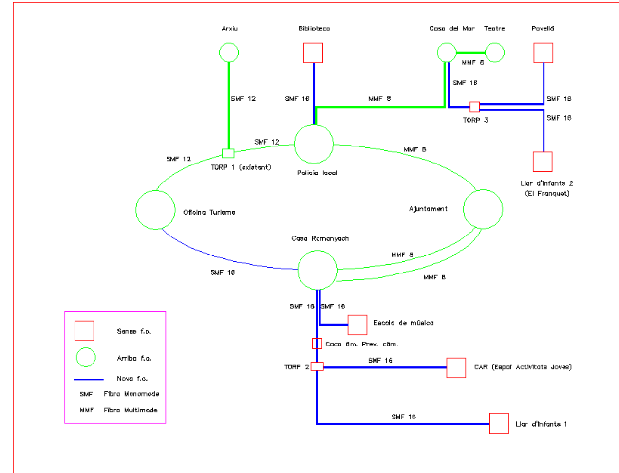
Esquema de la xarxa ampliada
