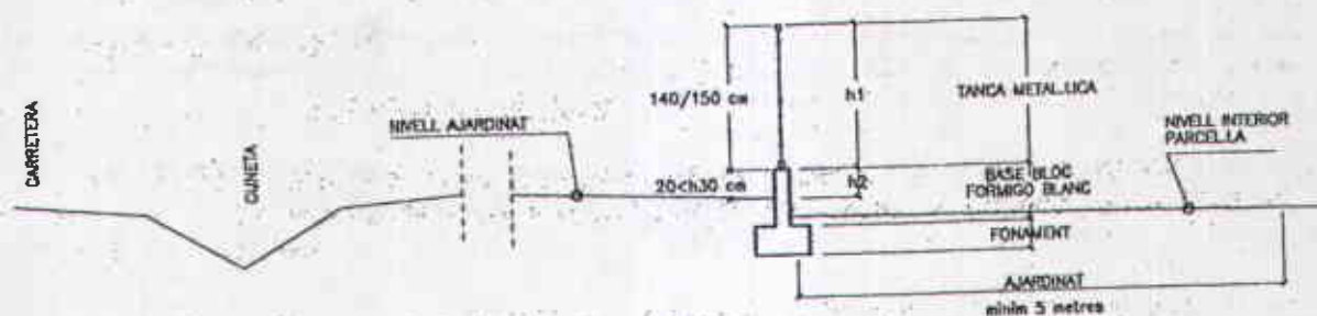
SECCIO CARRETERA
