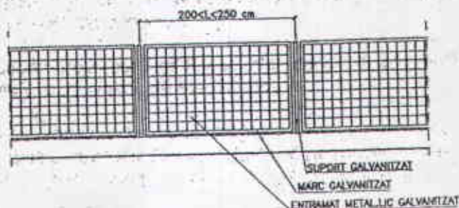
ALÇAT
