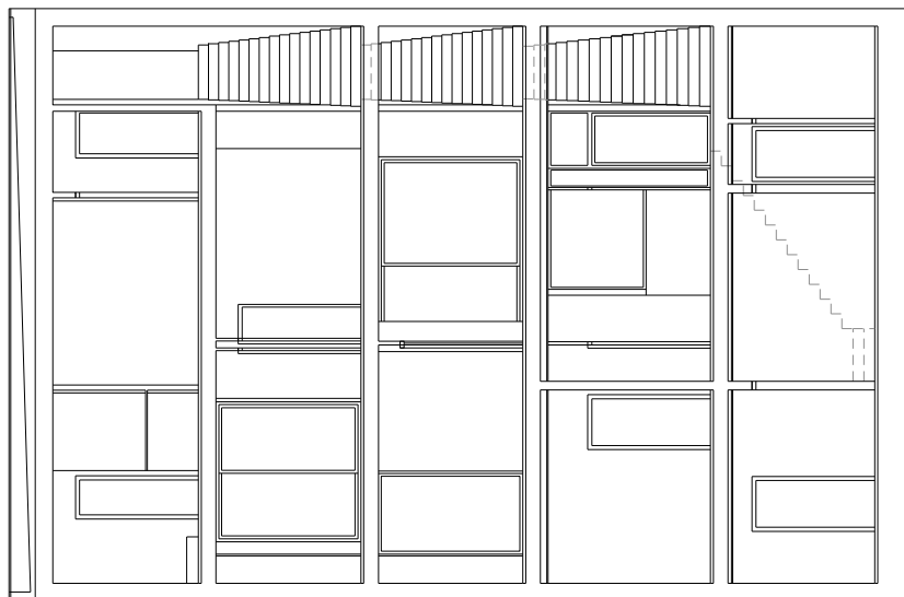
SECCIÓ A-A'
