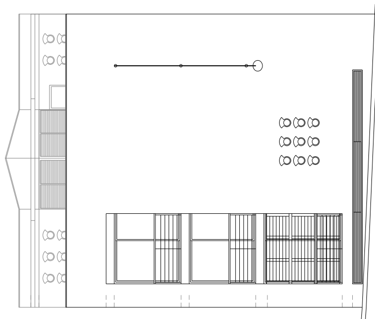
FAÇANA SUD-OEST (carrer de l'Escorxador)
