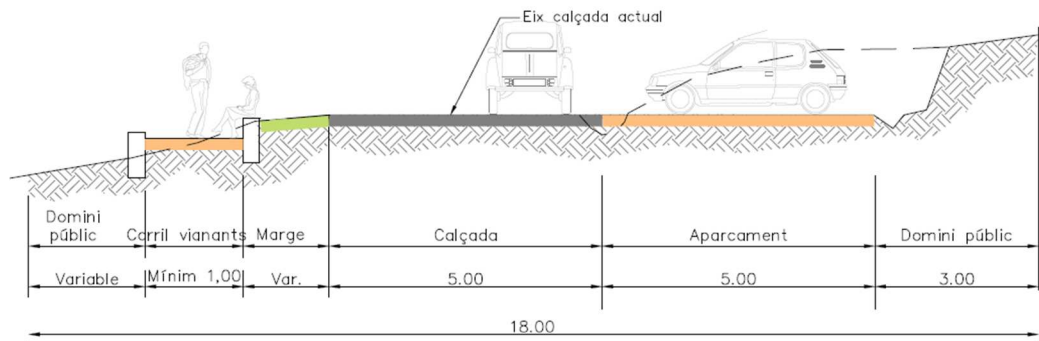
Secció D-D'
