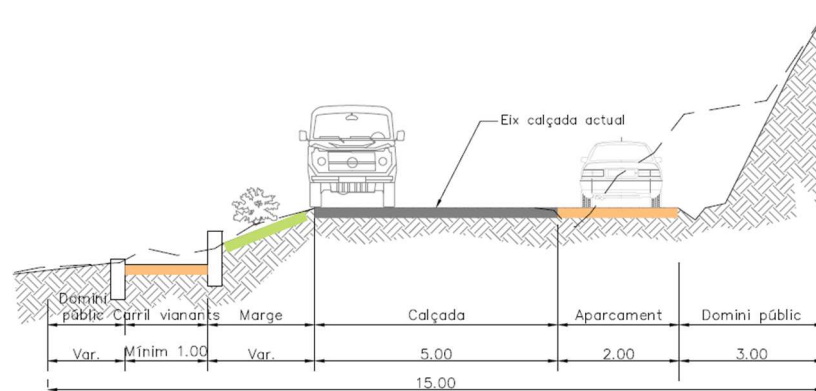
Secció C-C'
